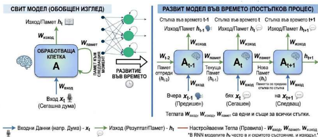
Фигура 28. Рекурентна невронна мрежа (RNN)
