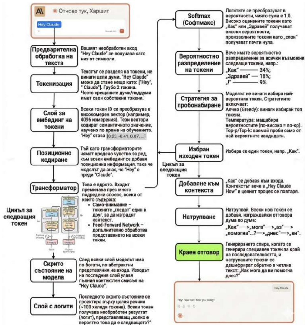
Фигура 46. Как работи Claude
