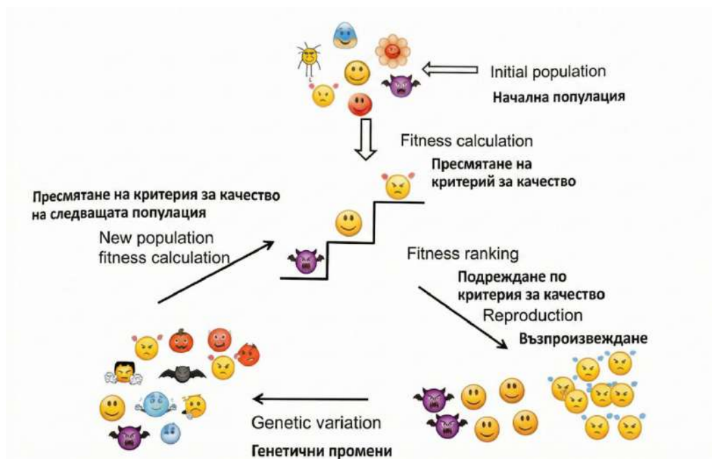
Фигура 38. Пример за работата на генетичен алгоритъм. 14
