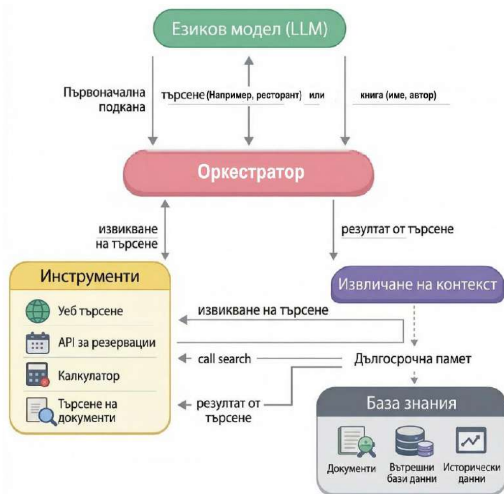
Фигура 62. Процес на работа на агента
