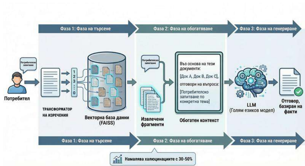
Фигура 50. Работа на Retrieval-Augmented Generation – RAG система
