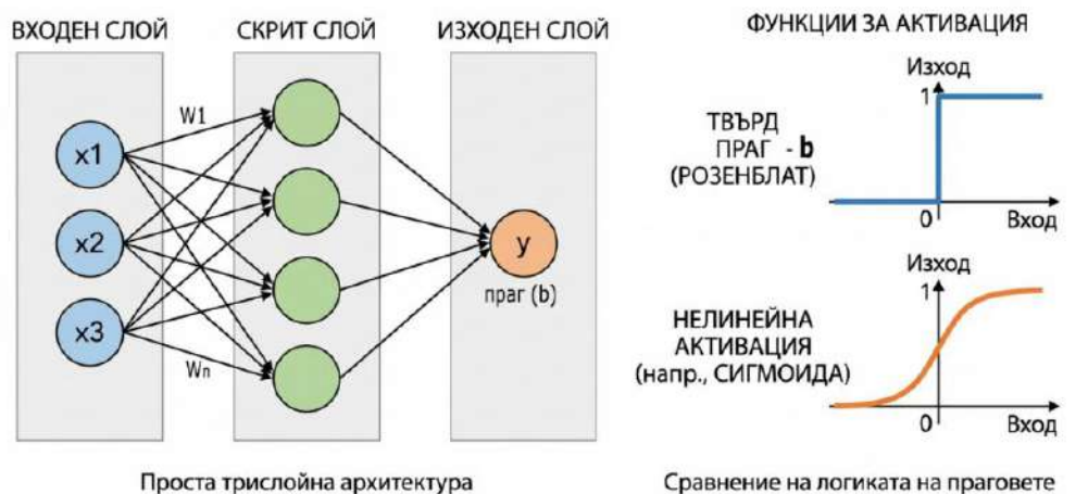
Фигура 25. Структура на изкуствена невронна мрежа (Перцептрон)
