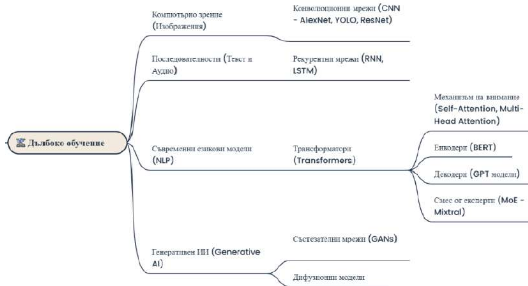
Фигура 26. Алгоритми за дълбоко обучение
