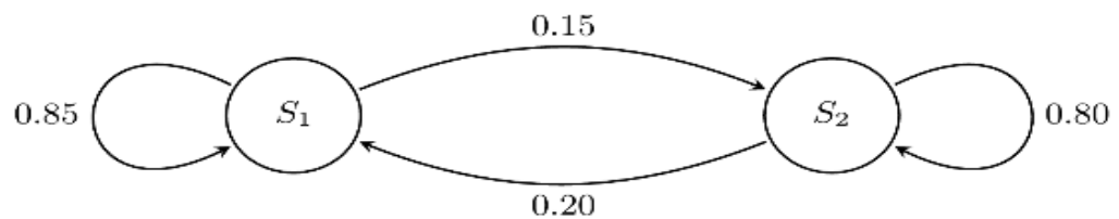
Фигура 23. Верига на Марков
