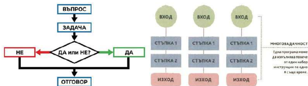
Фигура 33. Алгоритъм
