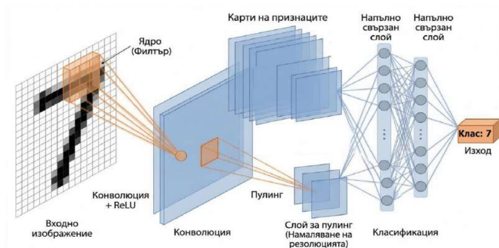
Фигура 27. Конволюционна невронна мрежа (CNN)
