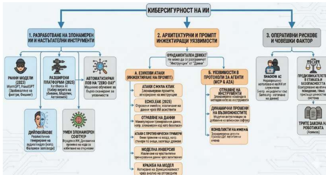
Фигура 63. Класификация на уязвимостите на AI
