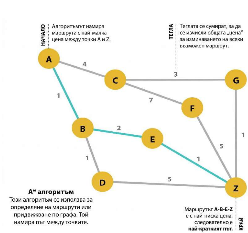
Фигура 41. Алгоритъм A* – намиране на най-кратък път
