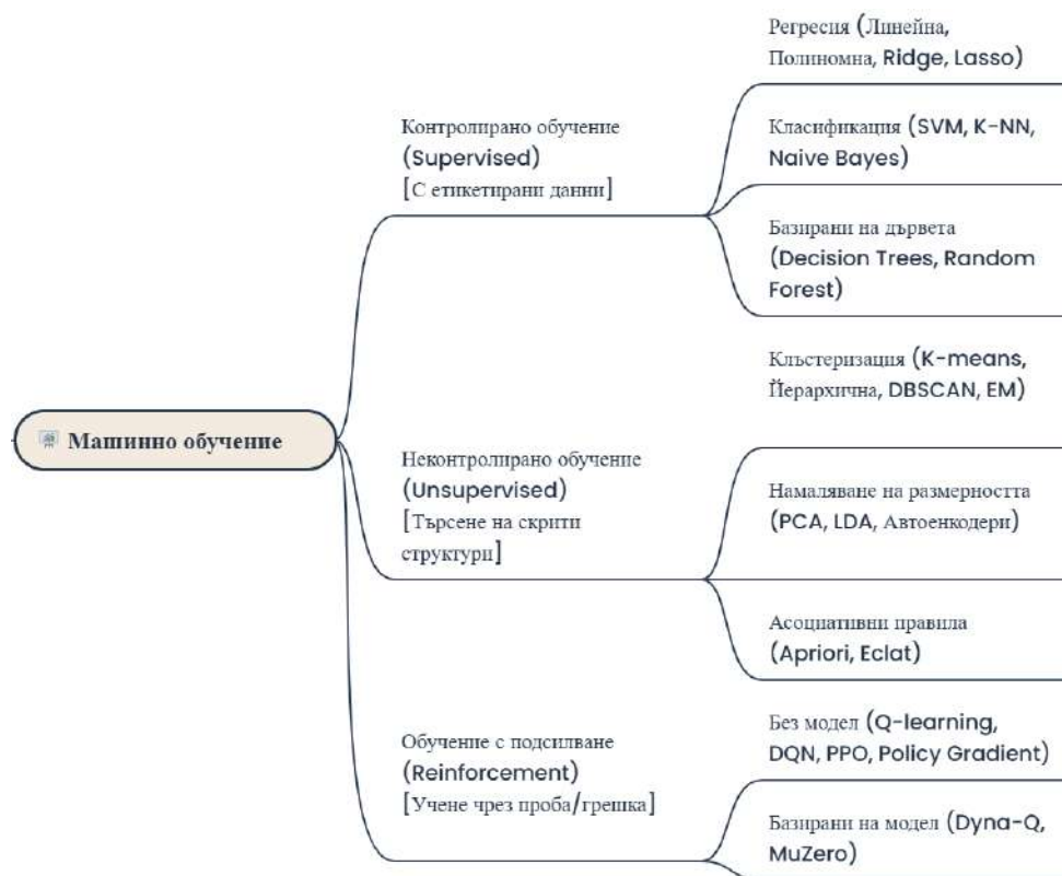
Фигура 18. Класификация на алгоритмите за машинно обучение
