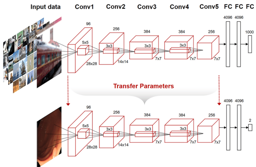
Фигура 10. Архитектура на AlexNet, базирана на няколко нива на невронни мрежи, означени с отделни блокове (conv1 – conv5) и три функционални нива (fc)
