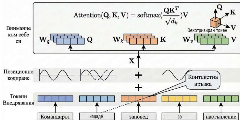
Фигура 44. Резултатът от softmax на вниманието към себе си
