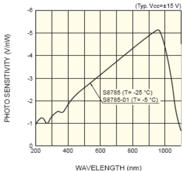
Фиг. 2. Спектрална характеристика на прибора
