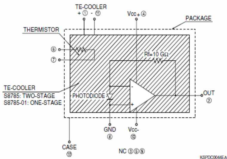
Фиг.1. Блокова схема на фотодиода с усилвател S8785 на един чип
