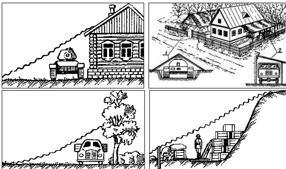
Фиг. 13. Маски навеси, използвани в зависимост от средата
