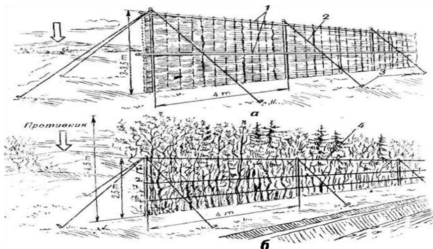
Фиг. 12. Вертикални крайпътни маски (1 – прътове; 2 – тел; 3 – колчета, 4 – обтегачи с два реда тел с диаметър 3 мм): а) с платна от сламени (пръти, камъш) рогозки; б) с платно от отсечени клони
