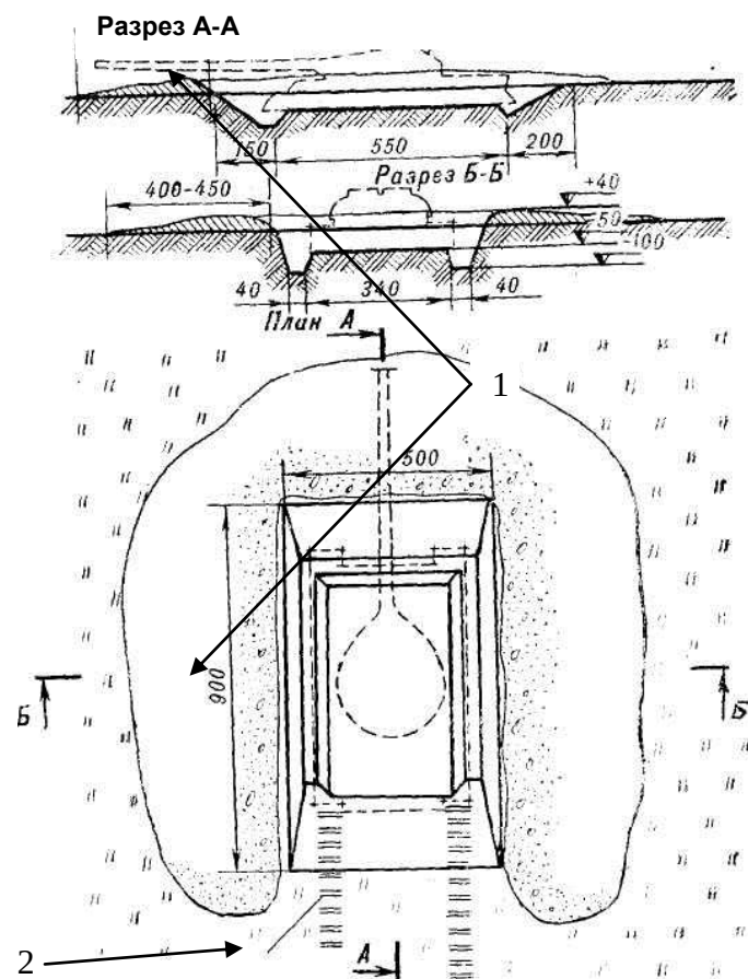
Фиг. 15. Лъжлив окоп за танк: 1 — контур на макета на танка, 2 — следи от вериги
